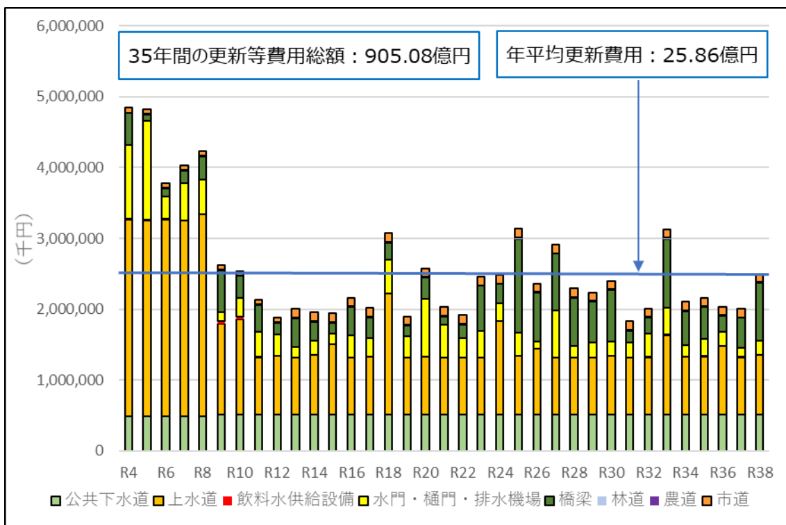
図表3-4：都市基盤施設に係る更新等費用の推計（対策前）
