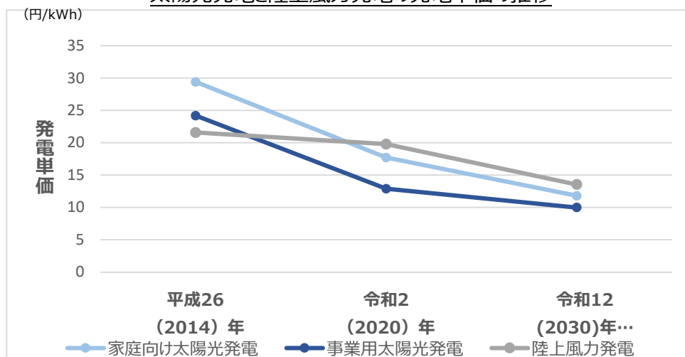
太陽光発電と陸上風力発電の発電単価の推移
