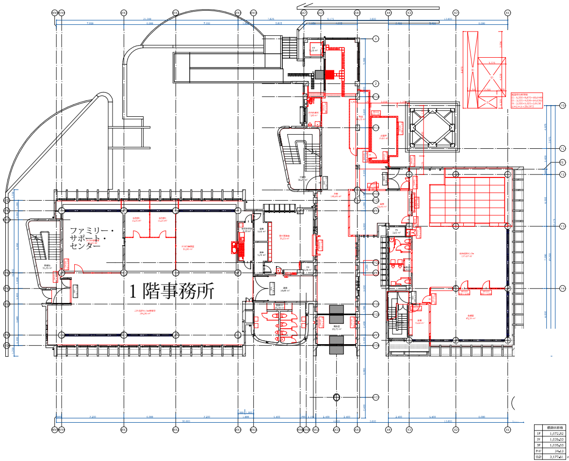
(仕様書別紙) 鳴門市こども未来館平面図 1階
