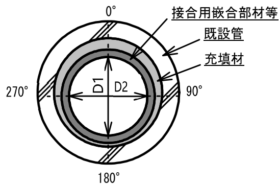
図 5.1.1 仕上り内径の測定位置(複合管)
