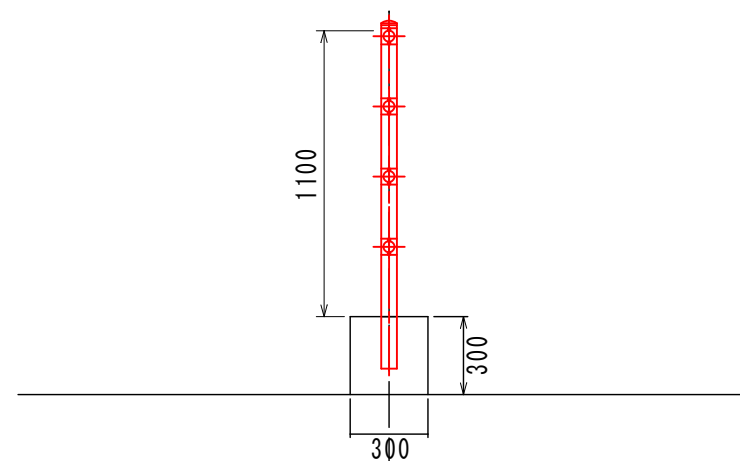
基礎横断面 S=1/30
