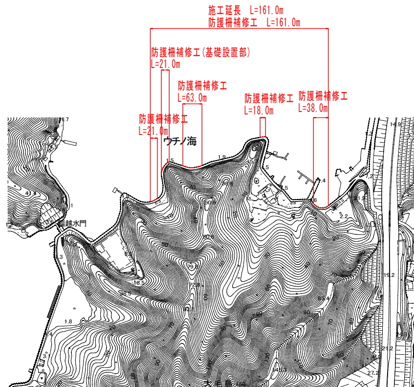
基礎縦断図 S=1/200
